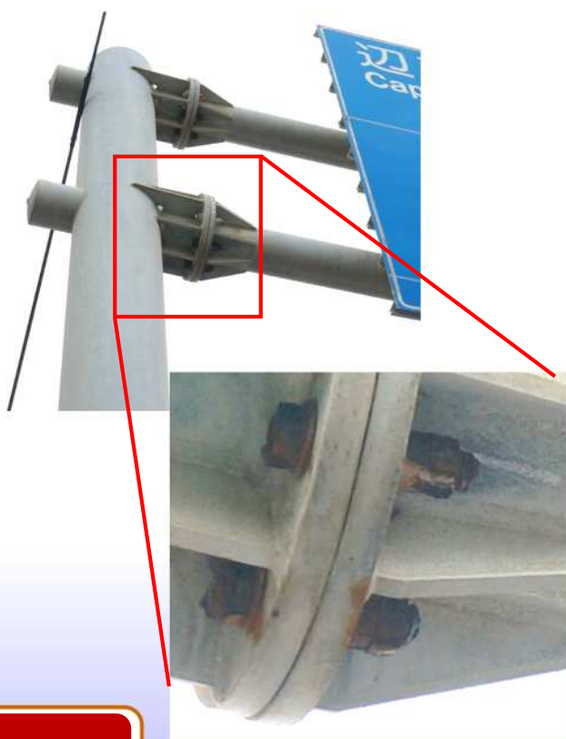
腐食ボルト
